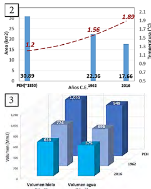
Fig. 1: Mapa de glaciares y paleoglaciares en la cuenca Parón, en líneas se muestra el cálculo de las ELA. Fig. 2: Variación del área vs. la variación de la temperatura. Fig. 3: Variación volumétrica de hielo y su equivalencia en agua.
